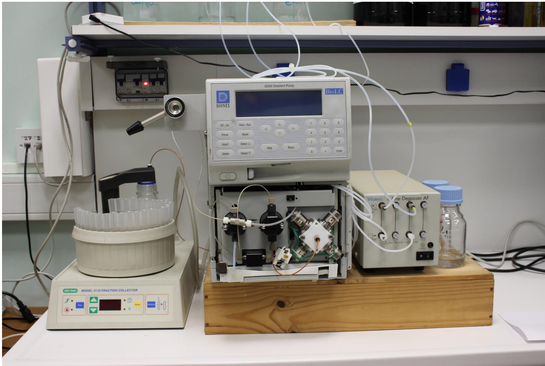
Υγροχρωματογράφος Dionex με συλλογέα κλασμάτων Bio Rad
