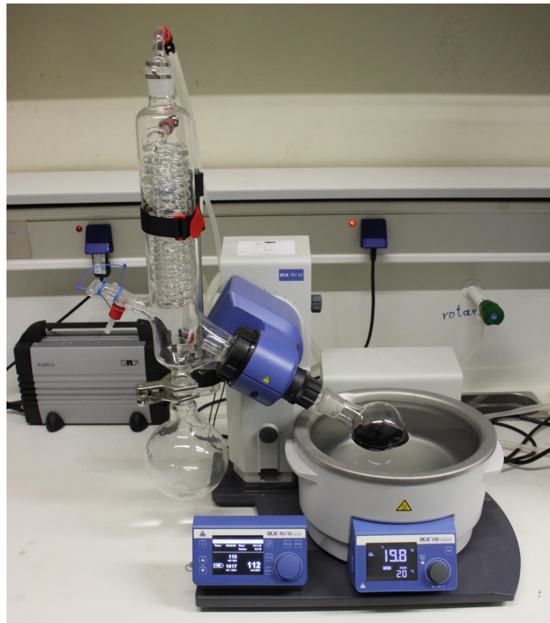
Περιστροφικός εξατμιστήρας IKA RV10 με αντλία κενού KNF N920G
