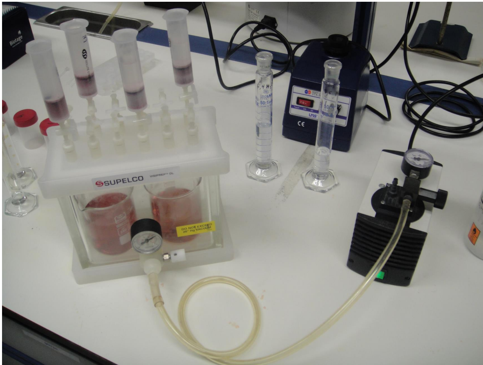
Συσκευή εκχύλισης στερεάς φάσης (Visiprep™ SPE Vacuum Manifold, Supelco)
